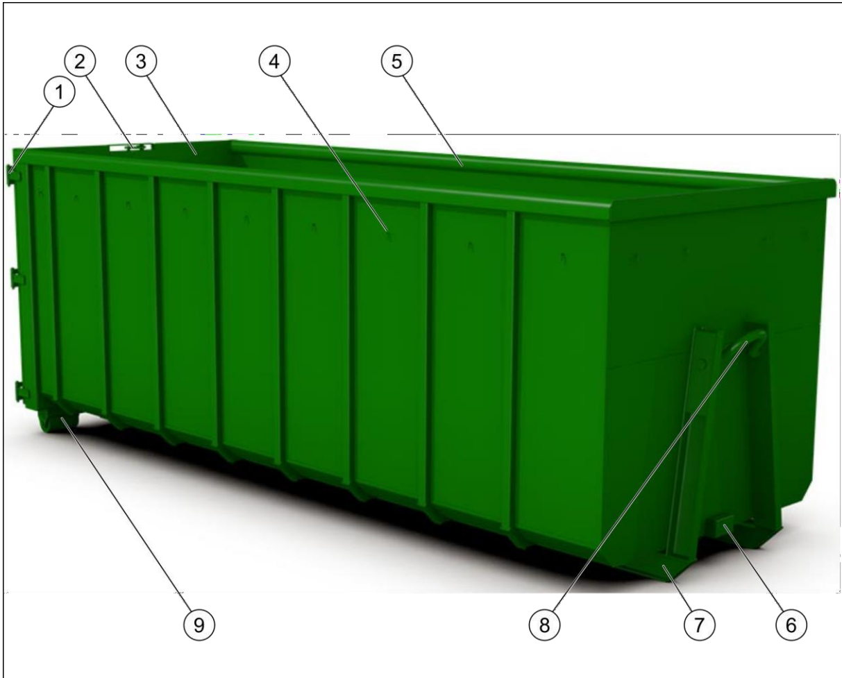
Abrollbehälter
